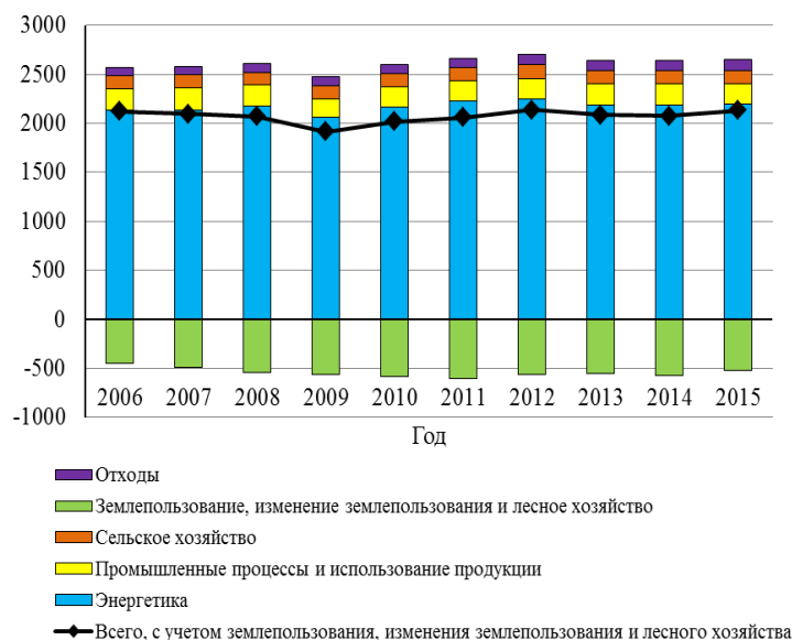
Рис. 4.1. Динамика выбросов парниковых газов в атмосферу, млн. т. CO 2 -экв.
