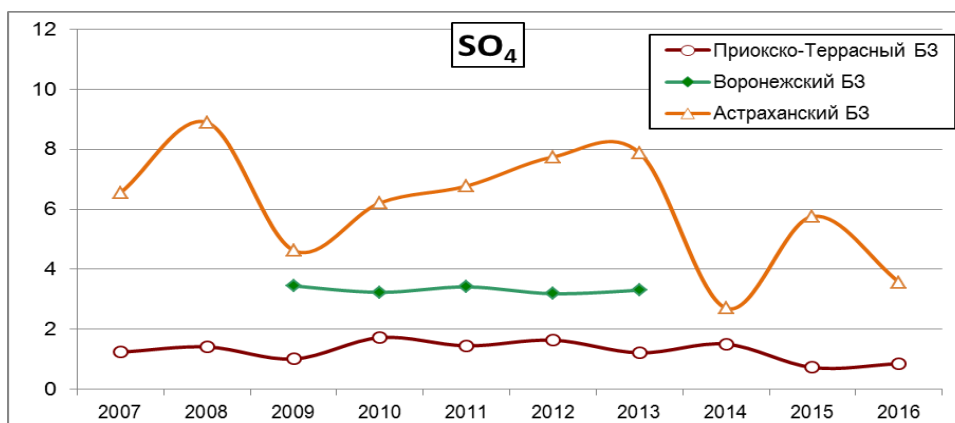
Рис. 5.2. Изменение фоновой концентрации диоксида серы, диоксида азота и сульфатов в атмосферном воздухе фоновых районов (мкг/м 3 )
