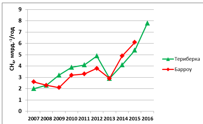
Рис. 5.1. Изменение скорости роста CH 4 с 2007 по 2016 гг.
