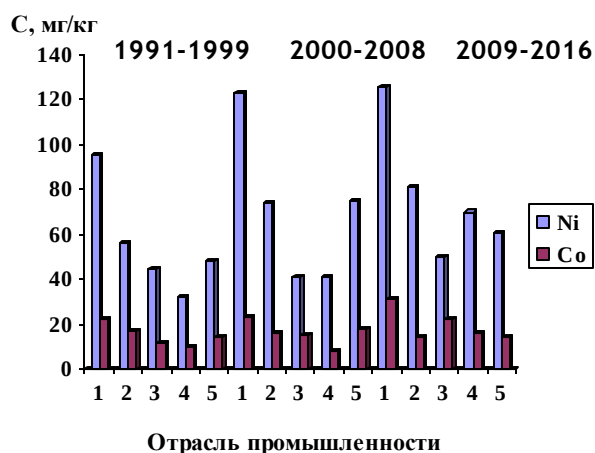
Рис. 6.7. Динамика средних по отраслям промышленности массовых долей, усредненных за определенные периоды: а) свинца и меди, б) никеля и кобальта в почвах 5-километровых зон вокруг предприятий металлургической промышленности (1), машиностроения и металлообработки (2), топливной и энергетической промышленности (3), химической и нефтехимической промышленности (4), строительной промышленности и производства стройматериалов (5)
