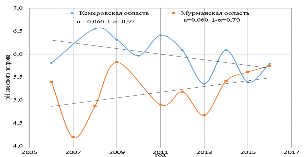
Рис. 5.8 (а). Линейные тренды изменения рН снежного покрова в Мурманской и Кемеровской областях за 2006-2016 гг.
