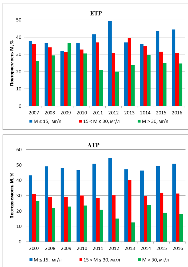
Рис. 5.4. Повторяемость минерализации осадков М (%) по градациям на ЕТР и АТР, 2007-2016 гг.
