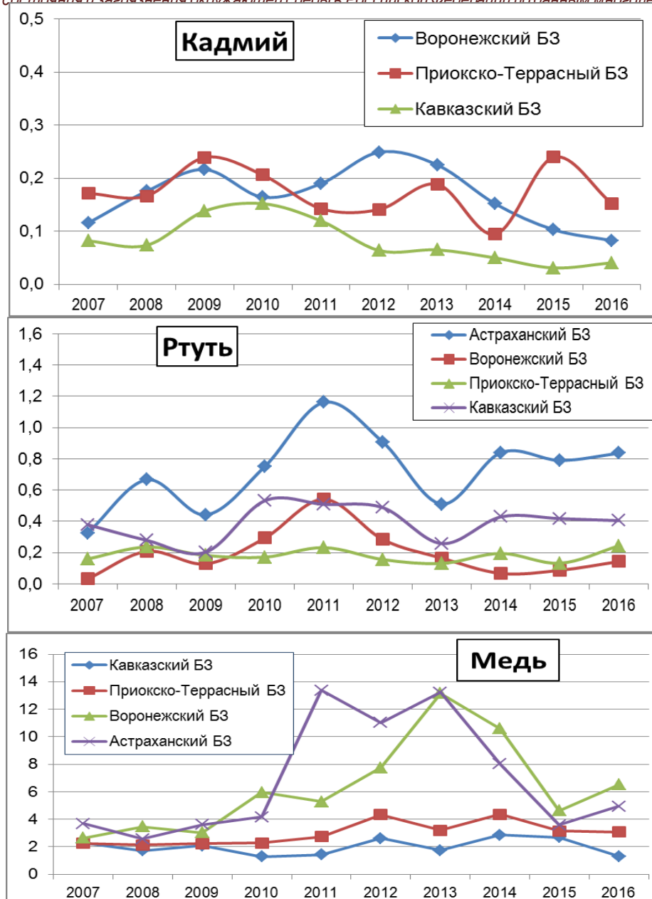
Рис. 5.13. Концентрации тяжелых металлов (мкг/л) в атмосферных осадках фоновых районов в 2006-2016 гг.
