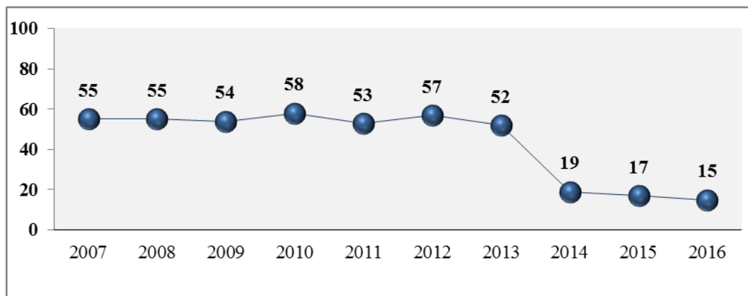
Рис. 6.5. Численность городского населения, %, испытывающего воздействие высокого и очень высокого загрязнения воздуха за период 2007-2016 гг.
