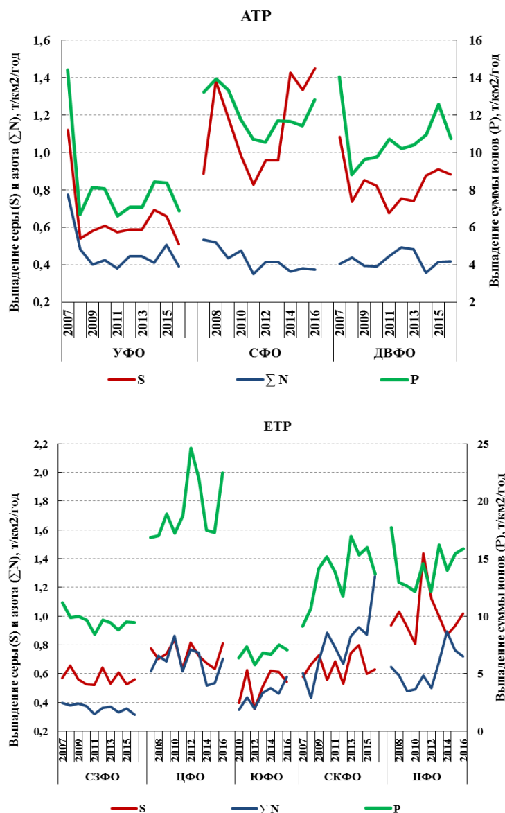
Рис. 5.6. Изменение влажных выпадений серы, суммарного азота и суммы ионов со временем по Федеральным округам на ЕТР и АТР, 2007-2016 гг.
