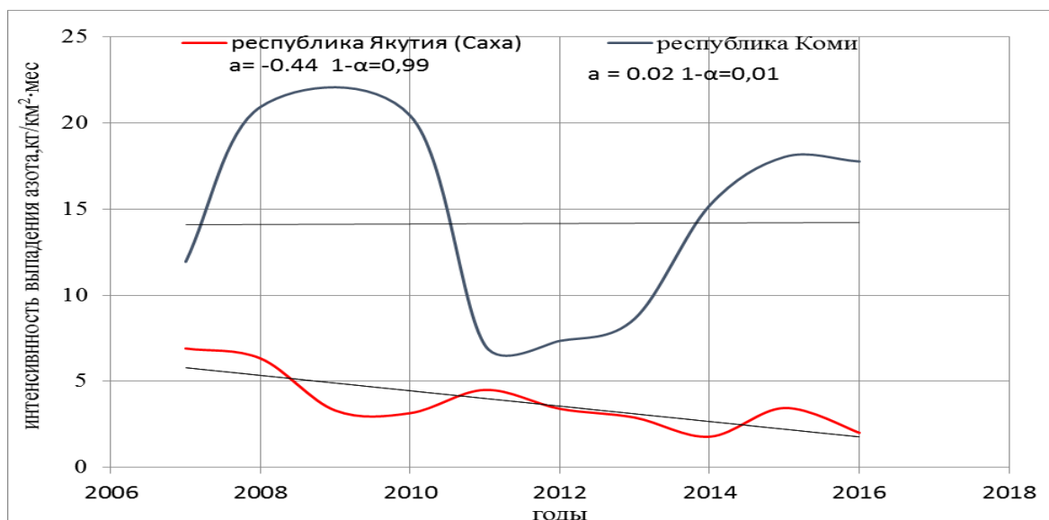
Рис. 5.12 (б) Линейные тренды изменения средней интенсивности выпадения азота I_N в зимние периоды в Республике Коми. и Республике Саха (Якутия) в 2007-2016 гг.
