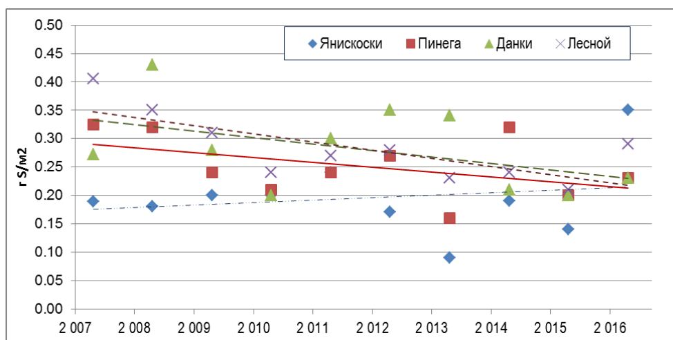
Рис. 5.15. Динамика ежегодных выпадений сульфатной серы из атмосферы с осадками на станциях ЕМЕП ( \text{г S/м}^2/\text{год} )
