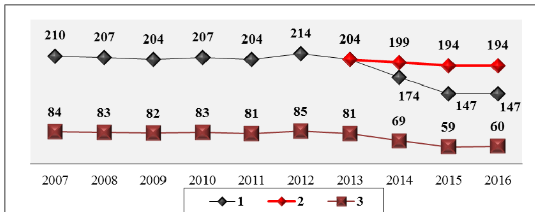
Рис. 6.3. Количество городов РФ, в которых среднегодовые концентрации одного или нескольких веществ превышали 1 ПДК, с учетом прежней и новой ПДК формальдегида и фенола (1, 2) и доля городов, %, в общем числе городов, где проводятся регулярные наблюдения (3) за период 2007-2016 гг.
