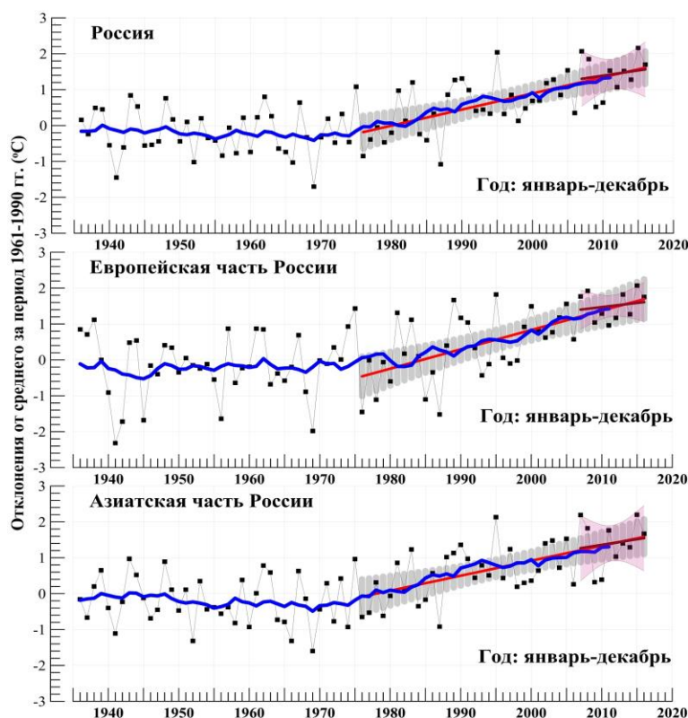
Рис. 1.1. Средняя годовая аномалия приповерхностной температуры России, ее европейской и азиатской части за 1936-2016 гг.
