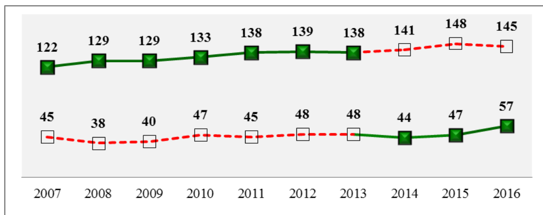
Рис. 6.6. Количество городов, в которых среднегодовые концентрации формальдегида превышают прежнюю (верхний ряд значений) и новую (нижний ряд) ПДКс.с. за период 2007-2016 гг.
