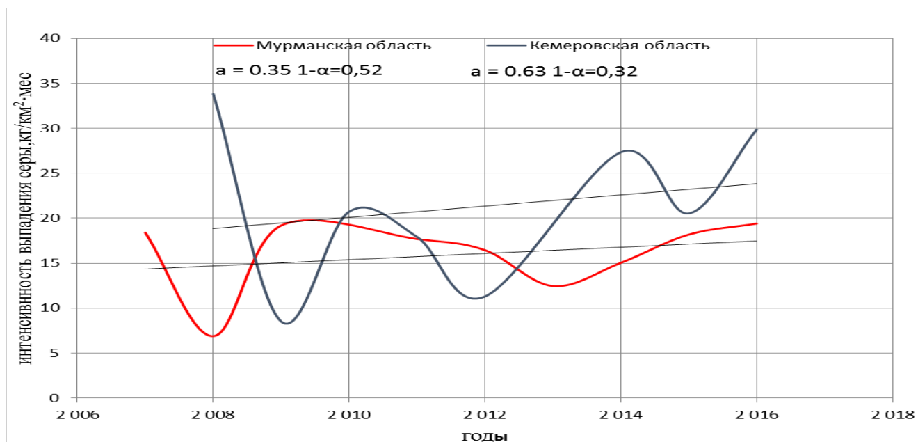
Рис. 5.10 (а) Линейные тренды изменения средней по площади региона интенсивности выпадения серы I_S в зимние периоды в Мурманской и Кемеровской областях в 2007-2016 гг.
