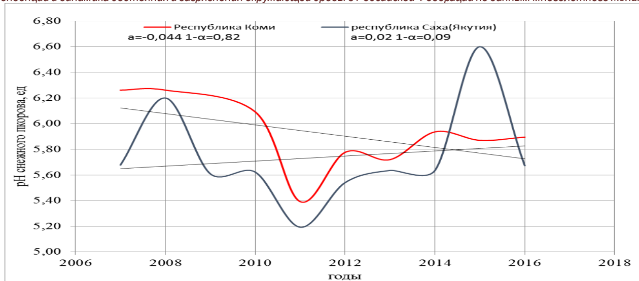
Рис. 5.8. (б). Линейные тренды изменения pH снежного покрова в Республике Коми и Саха (Якутия) за 2007-2016 гг.
