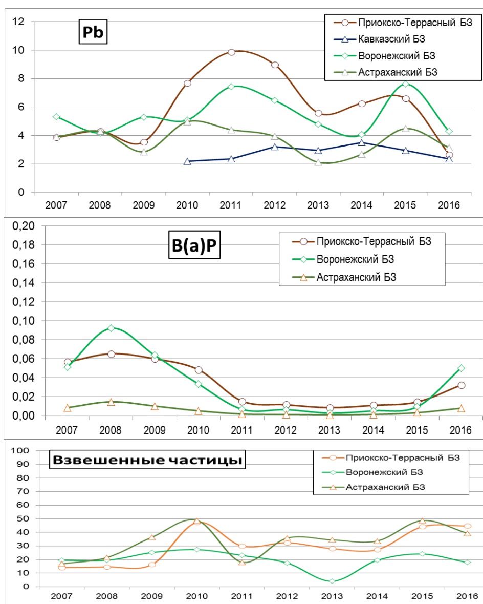
Рис. 5.3. Изменение фоновой концентрации свинца, 3,4-бензпирена (нг/м 3 ) и взвешенных частиц (мкг/м 3 ) в атмосферном воздухе фоновых районов.
