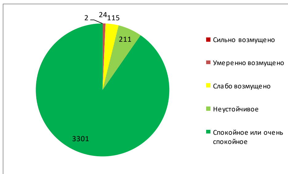
Рис. 2.3. Состояние магнитного поля Земли
