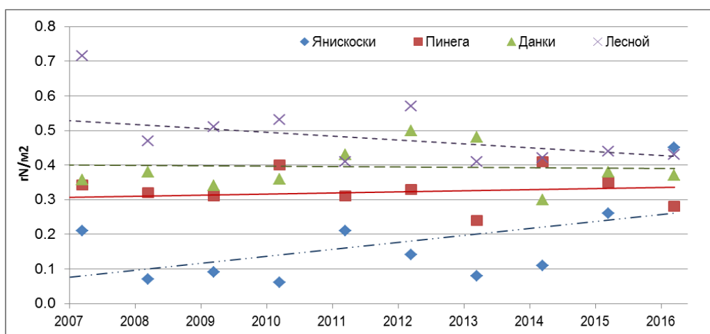
Рис. 5.16. Динамика ежегодных выпадений суммарного азота (нитратного и аммонийного) из атмосферы с осадками на станциях ЕМЕП ( \text{г N/м}^2/\text{год} )
