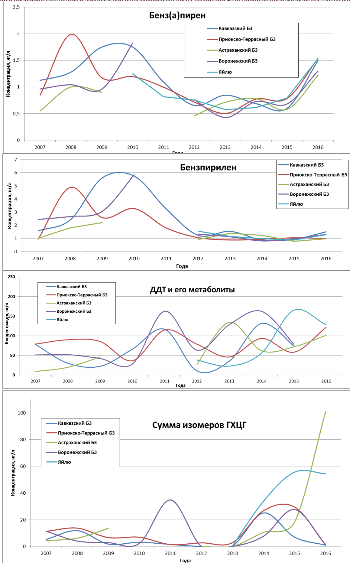
Рис. 5.14. Концентрации полиароматических углеводородов и хлорорганических пестицидов (нг/л) в атмосферных осадках фоновых районов за период 2007-2016 гг.
